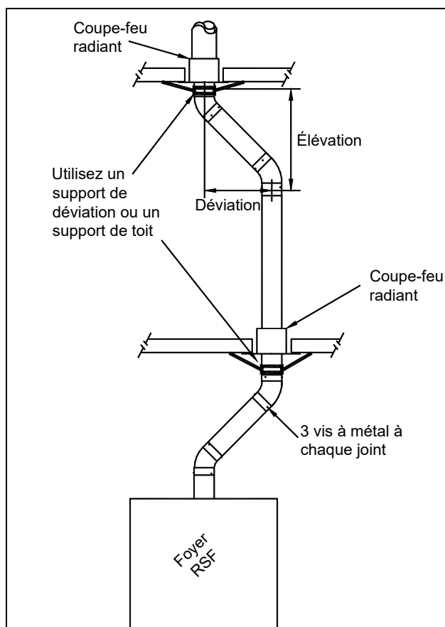
Figure 14 Exemple d'installation d'une cheminée avec déviation
