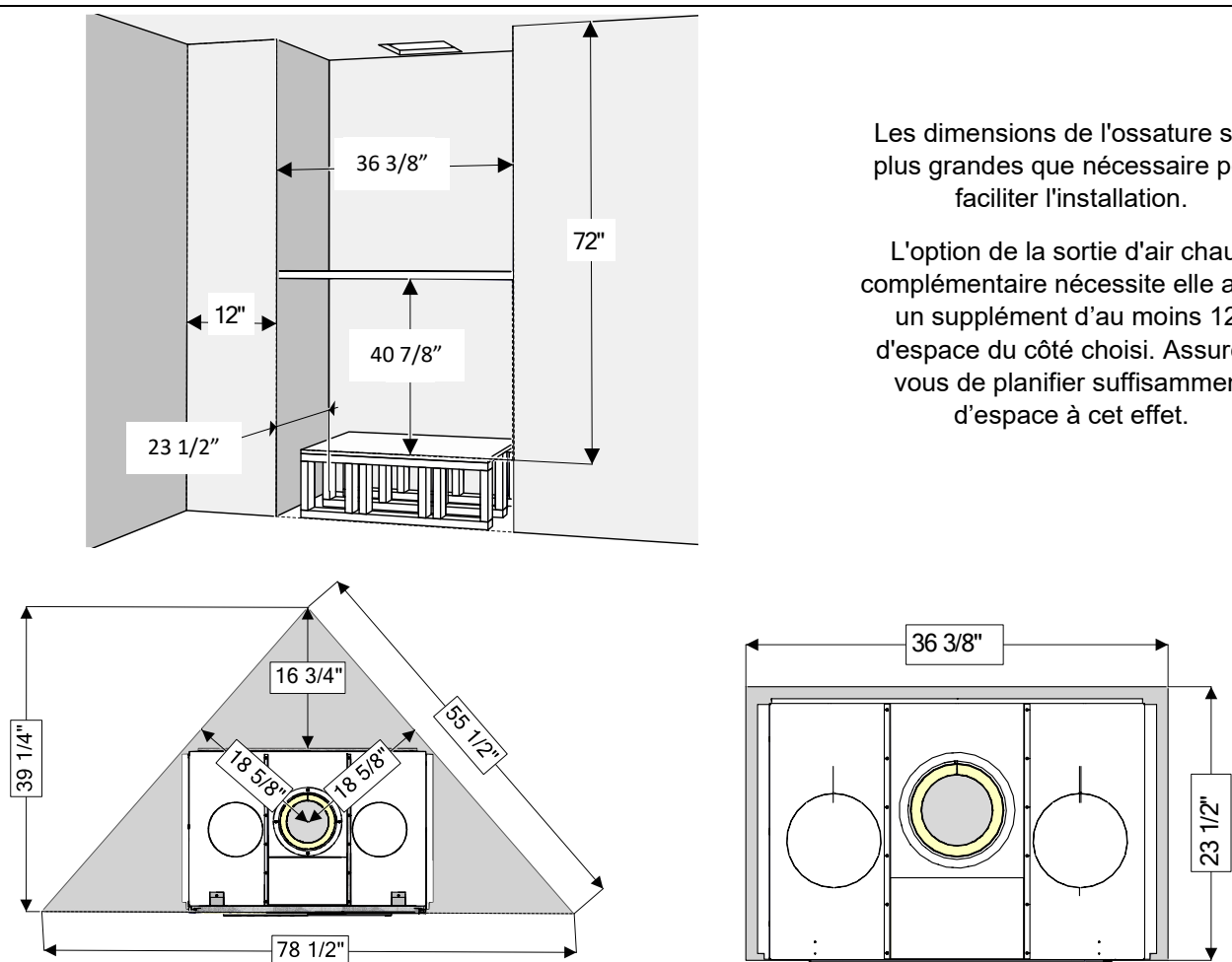
Figure 4 Exemples d'ossature pour le FOCUS 3600
