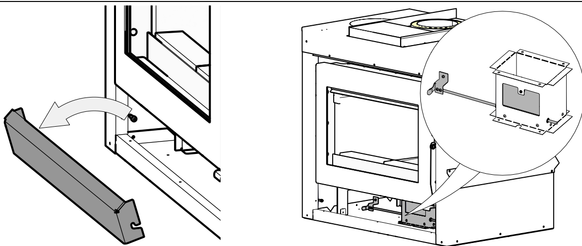
Figure 23 Emplacement du contrôle d'air extérieur
