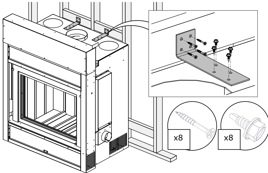
FIGURE 11 INSTALLATION DES SUPPORTS DE STABILITÉ ANTI-RENVERSEMENT
